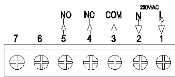
Šema povezivanja
